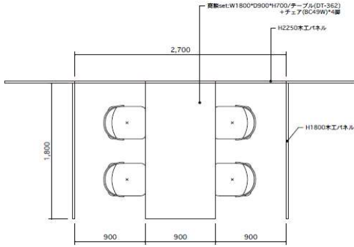
(平面図)
