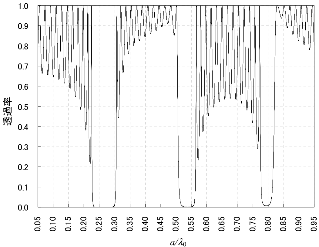
図 40-3 多層膜の透過率 ( n_L = 31 )
