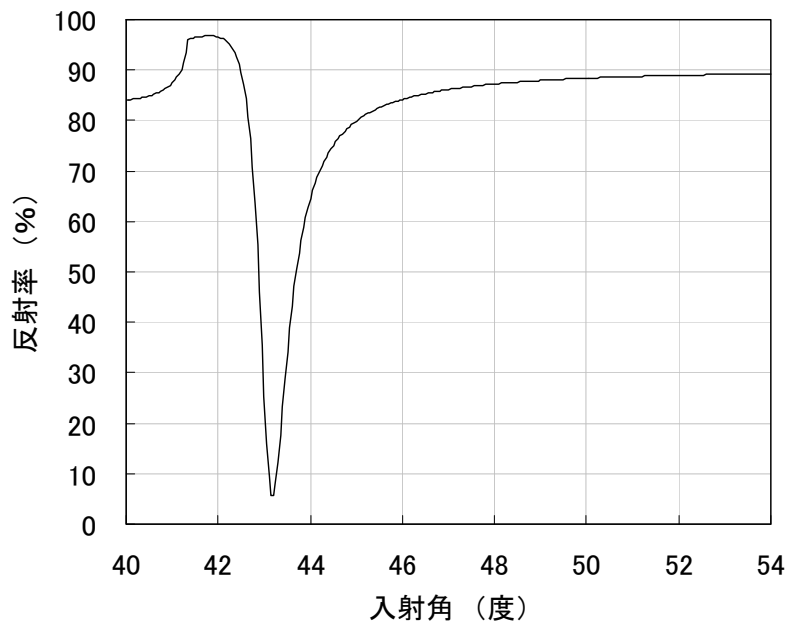
図 36-2 反射率の入射角依存性 鋭い表面プラズモン共鳴がある
