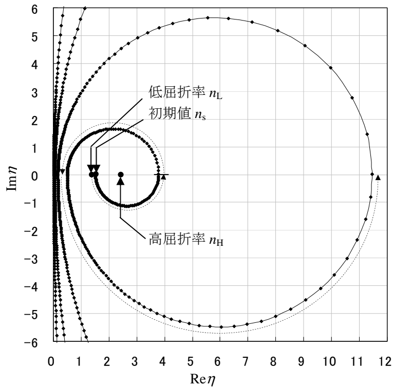
図 45-1 多層膜反射鏡 [n_0(\text{HL})^4\text{H}n_s] のアドミタンス軌跡 ( n_L = 1.38, n_H = 2.40, n_s = 1.52 )
